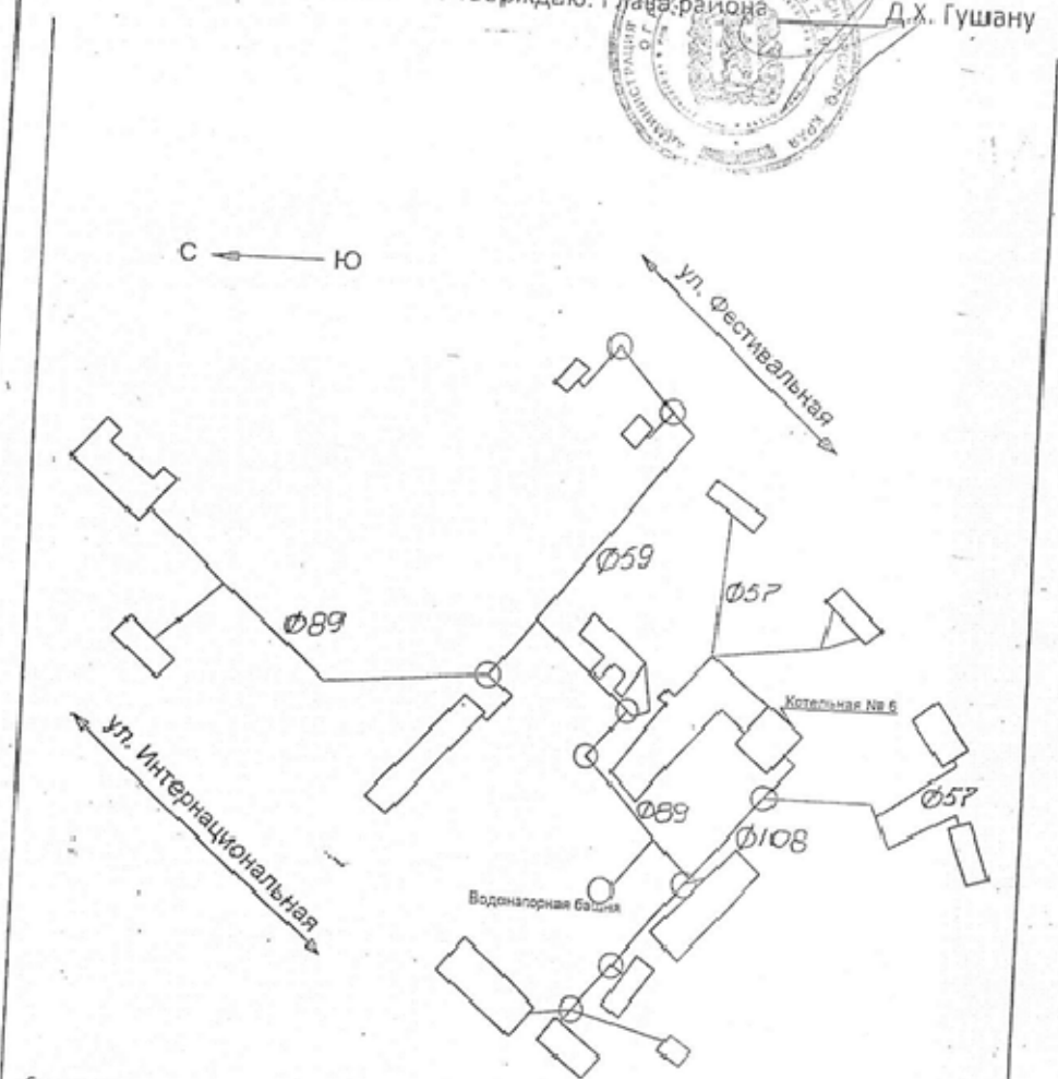
Схема прокладки тепловых и водопроводных сетей
