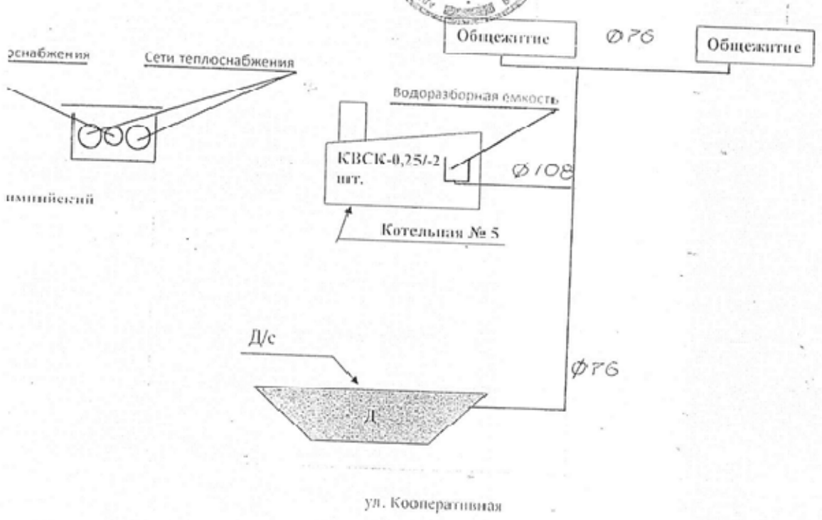
Рисунок 5 - Схема тепловой сети от котельной №5
